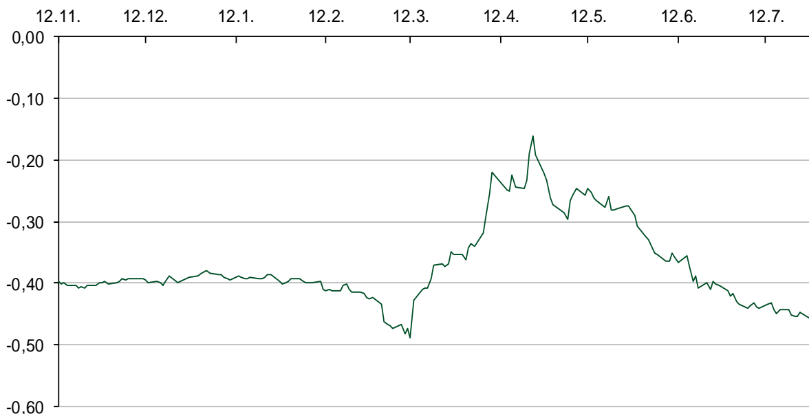
Euribor 3M
