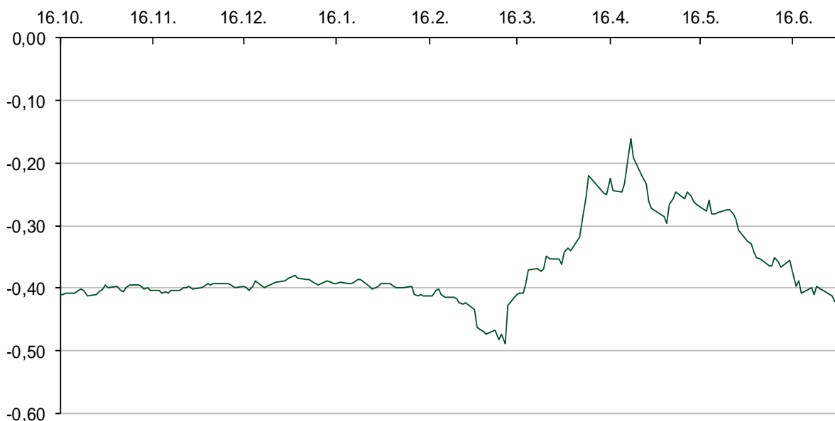
Euribor 3M
